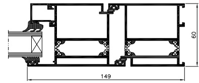
MB-60 Tür – Schnitt
