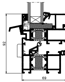
MB-60HI Fenster – Schnitt
